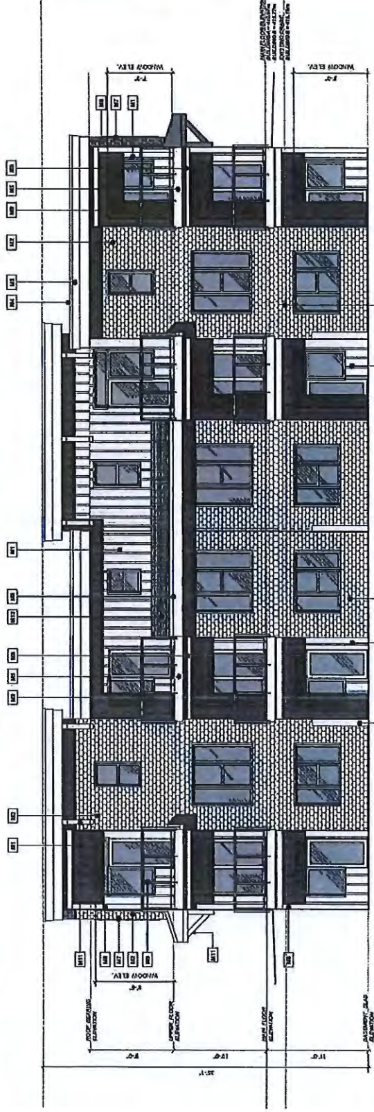
2 SIDE ELEVATION Scale: 1/8" = 1'-0"
